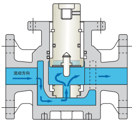
阀截面图
