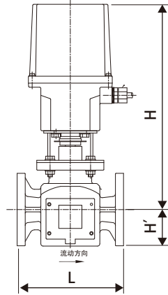
外形尺寸图
