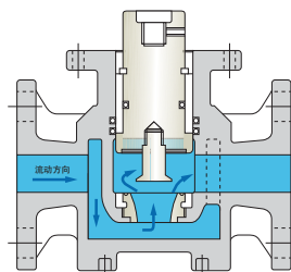
阀截面图
