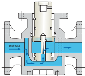
阀截面图
