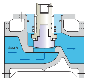
阀截面图
