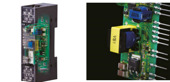
专为M5-UNIT设计的电子电路 M5VS的电路是以不影响性能、品质,将部件数量减至最少为宗旨设计的高效率电子电路。
