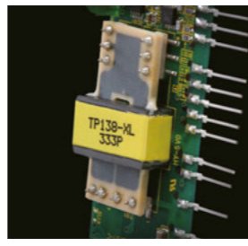
薄板式变压器 通过绕组线圈为印刷电路板结构的超薄型板式变压器,在不占空间的情况下实现了隔离强度2000V AC。
