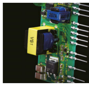
专为M5-UNIT设计的电子电路 M5VS的电路是以不影响性能、品质,将部件数量减至最少为宗旨设计的高效率电子电路。
