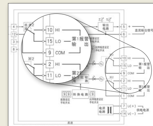
简易电路图
