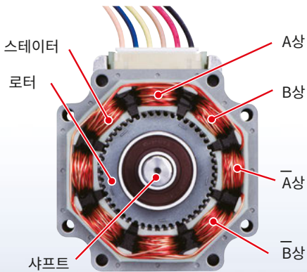
2상 8극 모터의 경우
