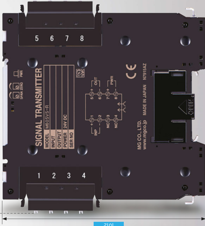
깊이 102 mm
