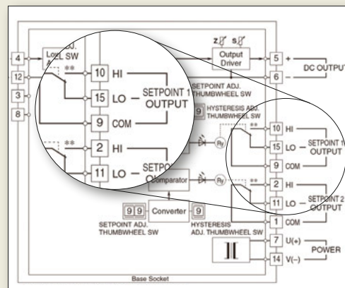
블록도
