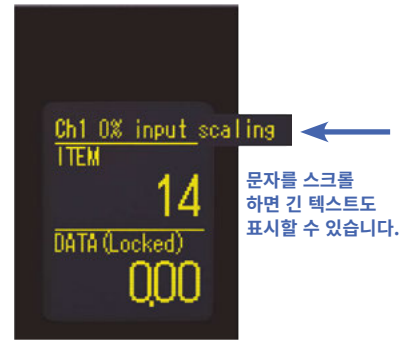
설정 화면
