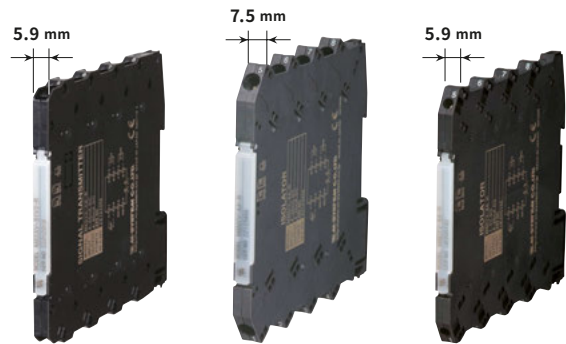
스프링식 단자 접속형 M6S 시리즈
