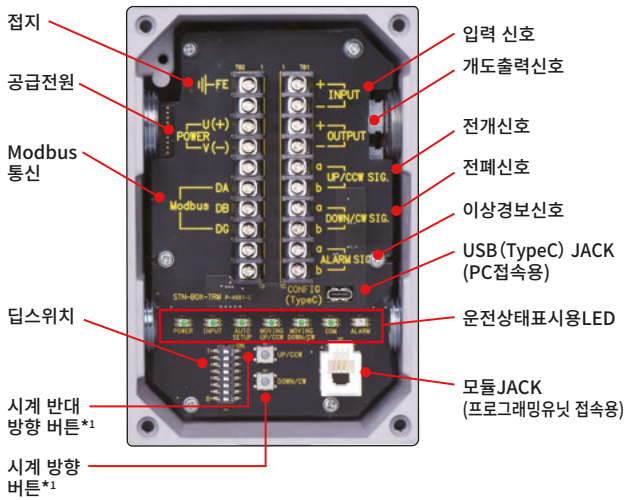
터미널박스
