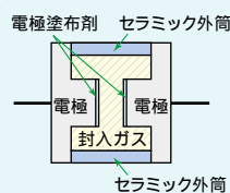
図2 放電管の断面図
