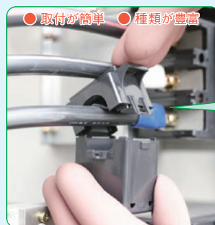
図1 クランプ式交流電流センサ
