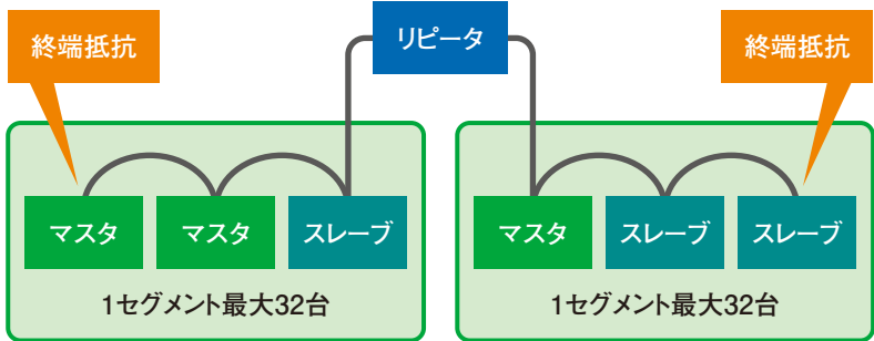
図1 BACnet MS/TP接続イメージ
