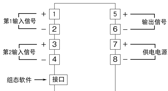
端子连接图
