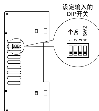
■右侧视图
