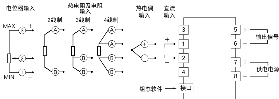
端子连接图
