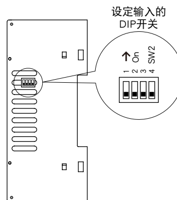
■右侧视图
