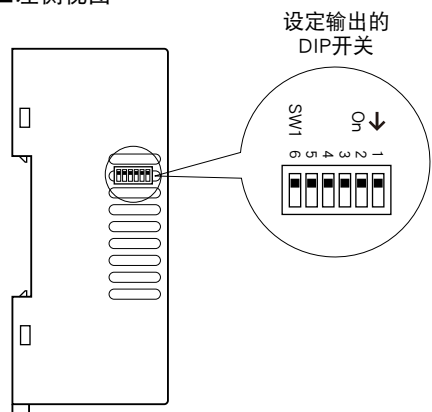
■左侧视图
