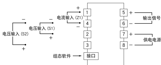
端子连接图
