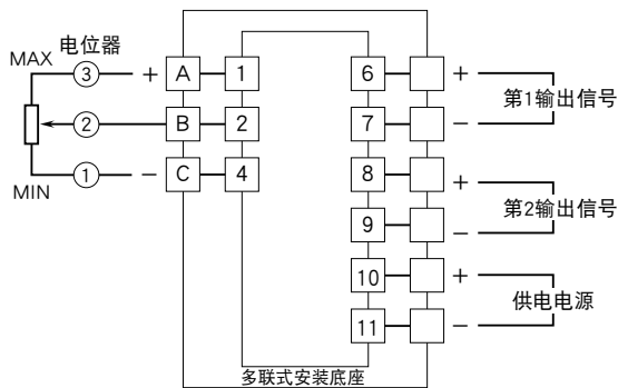
端子接线图
