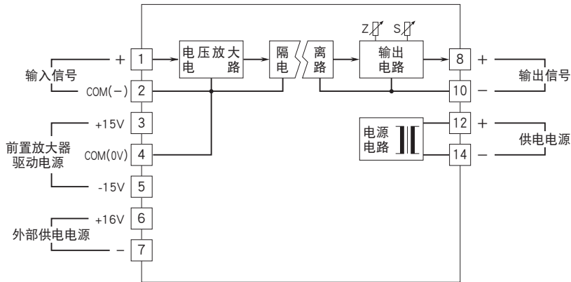
简易电路图 · 端子接线图
