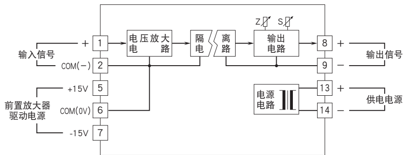
简易电路图 · 端子接线图
