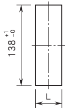
安装面板厚度:1.6~8.0 L = \{ 31.5 + 36 \times (N - 1) \} (N为连接数)
