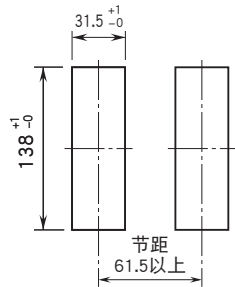
安装面板厚度:1.6~8.0
