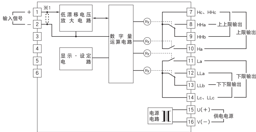
■ 48NDV-4 (4点报警/4个接点输出)
