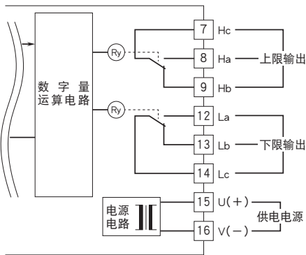
■ 48NDV-2 (2点报警/2个接点输出)
