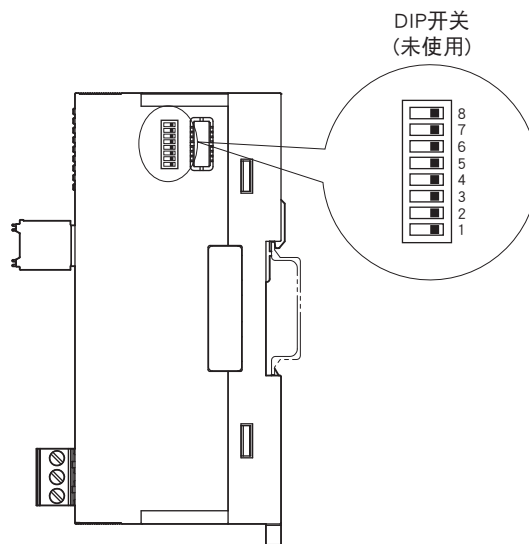
■ 侧视图
