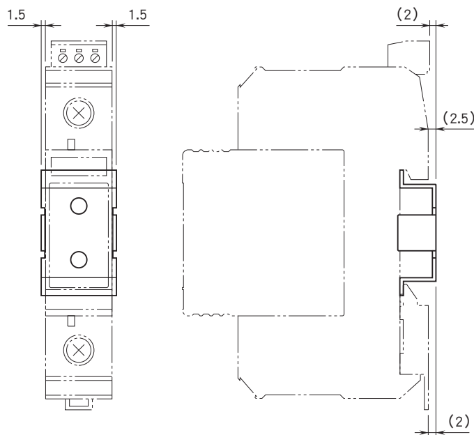
■MBS与避雷器的安装组合图
