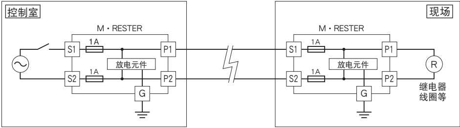
雷浪涌吸收元件断路时，为了使保险丝断开，布线时请将本产品的S1、S2端子接在供电侧。
