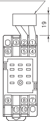
输入电阻器 (REM2)
