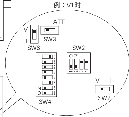
■左视图 (关闭前端面板盖时)
