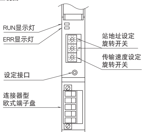
■正视图
