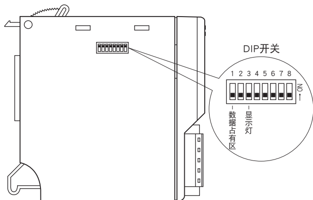
■左侧视图
