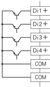
●接点输入连接例
