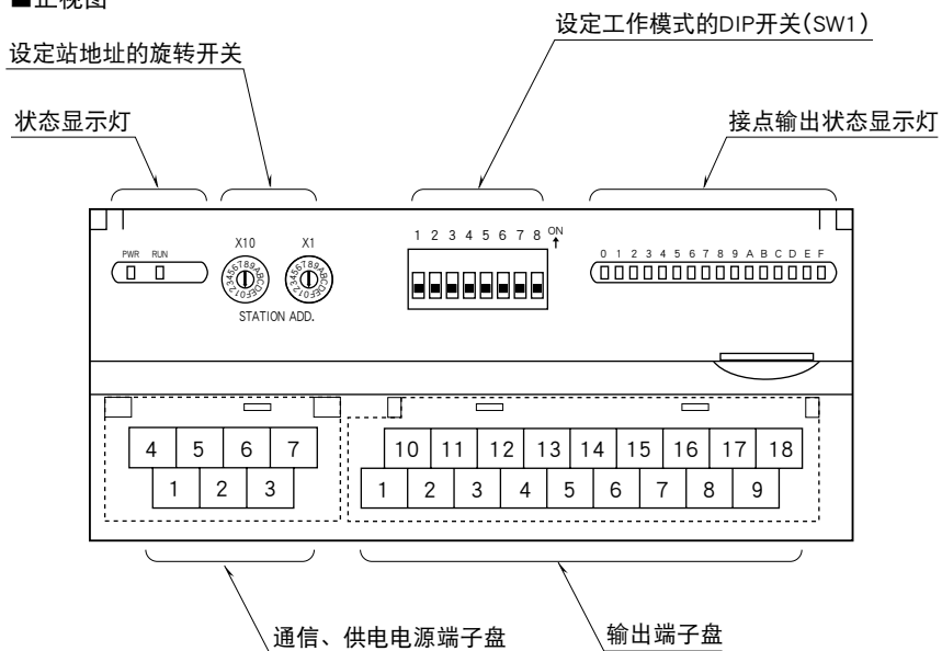
■正视图
