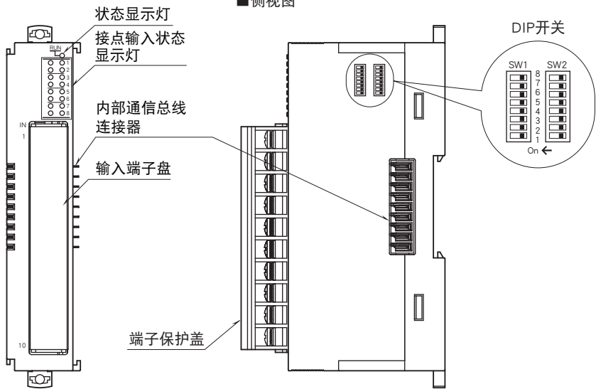
■ 侧视图
