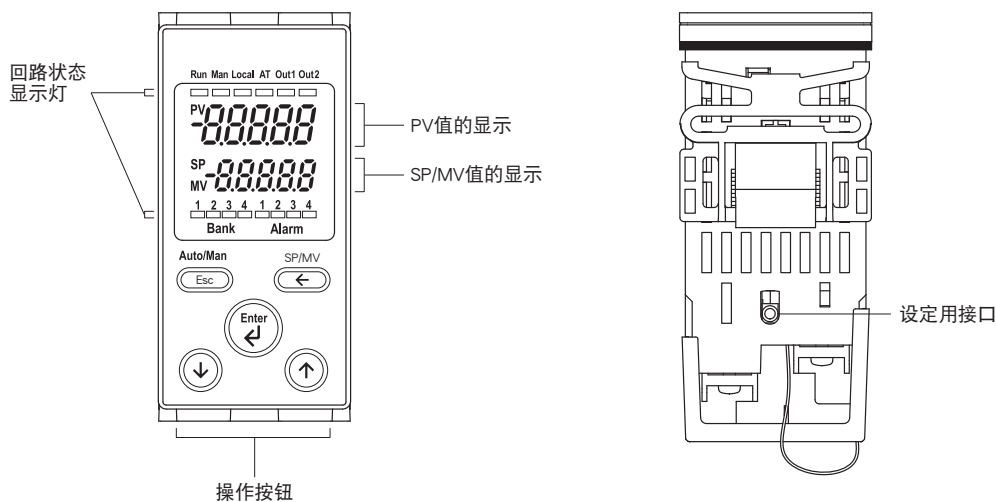
■正面图
