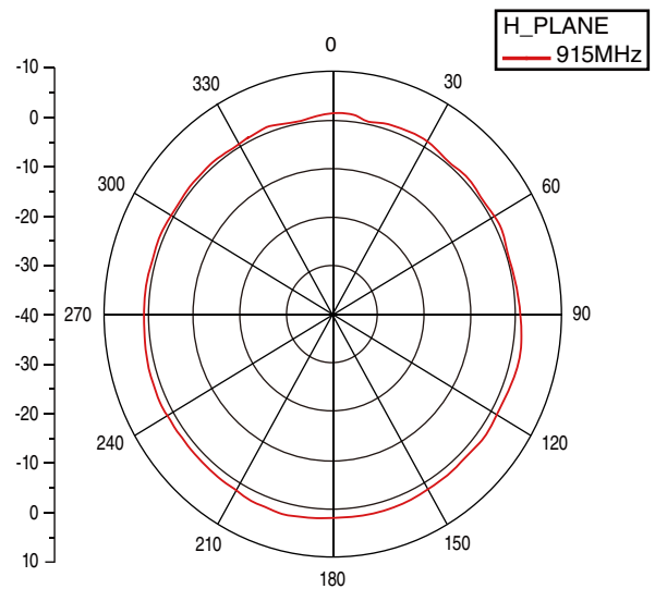
[H-Plane]
