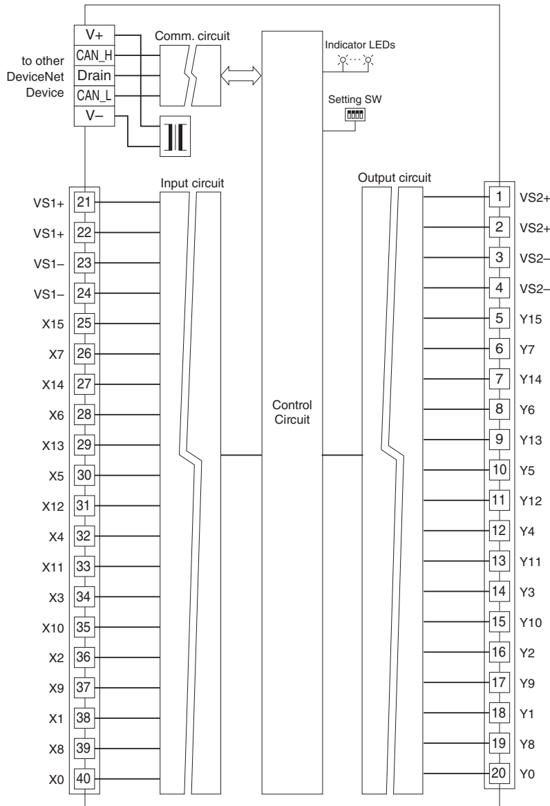
■ Input Circuit
