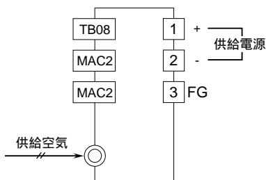
端子接続図
