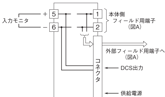
図A フィールド用端子接続図
