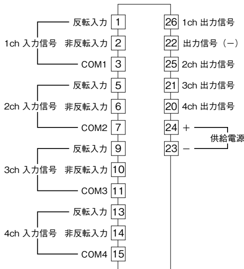
端子接続図
