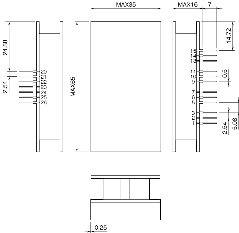
外形寸法図 (単位: mm) ・ 端子番号図
