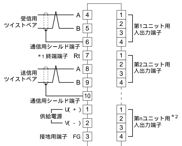
端子接続図
