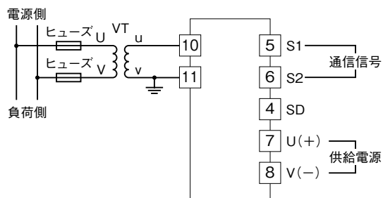
端子接続図
