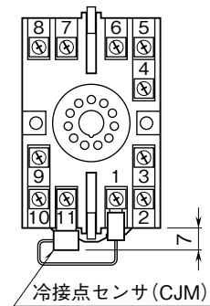
端子番号図 (単位: mm)
