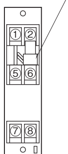
冷接点センサ (CJM)
