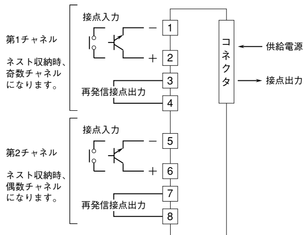
端子接続図
