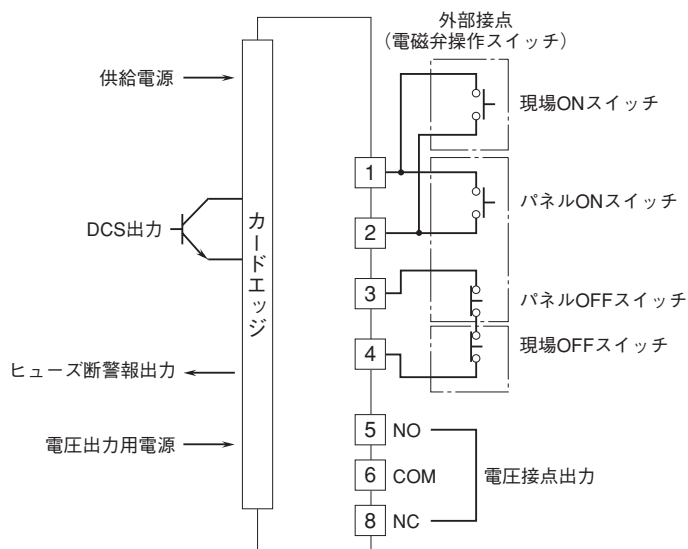
端子接続図
