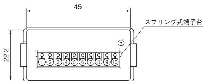
■背面図
