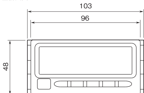
■前面図
