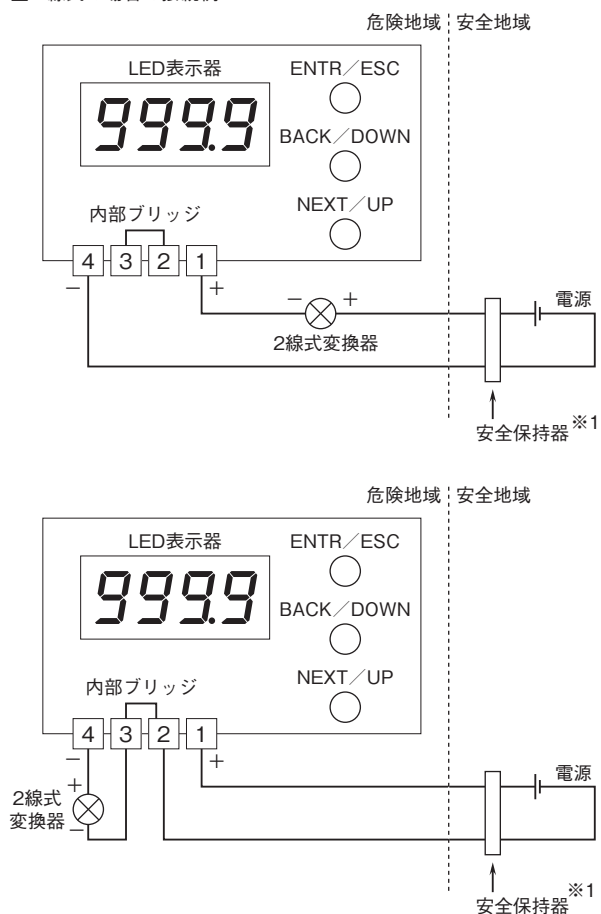
■2線式の場合の接続例
