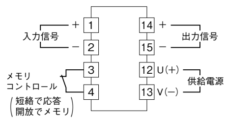
端子接続図
