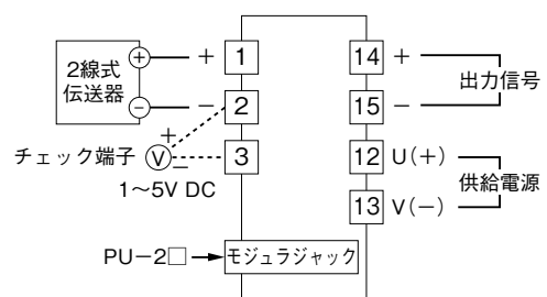
端子接続図
