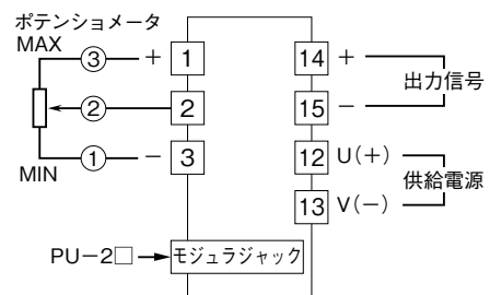
端子接続図
