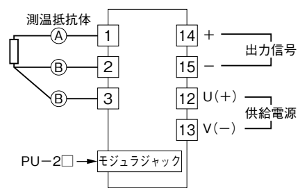
端子接続図
