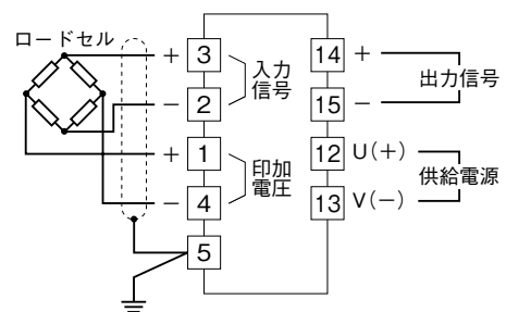
端子接続図
