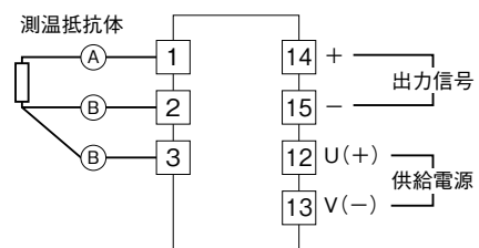
端子接続図
