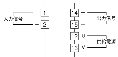
端子接続図
