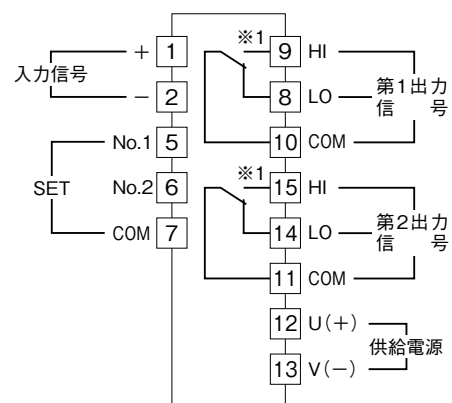
端子接続図
