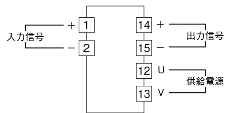
端子接続図
