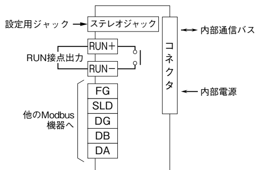
端子接続図
