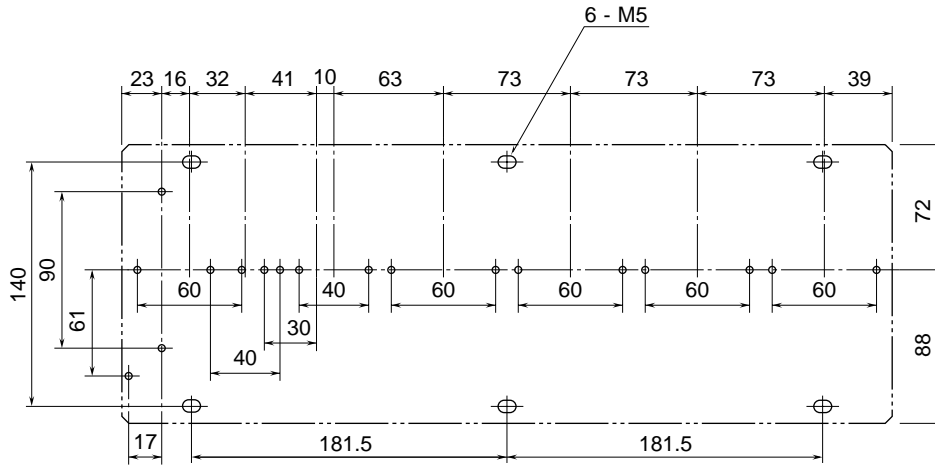
取付寸法図 (単位: mm)
