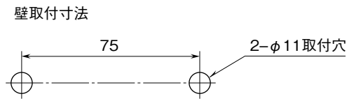
取付寸法図 (単位: mm)
